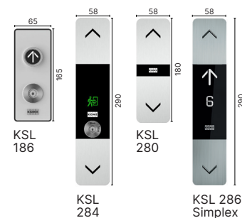
KONE Interact 10 Altezza totale** montaggio a filo
